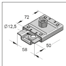
Element ślizgowy GL 37
